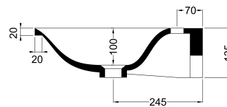
SEZIONE A-A SECTION A-A
