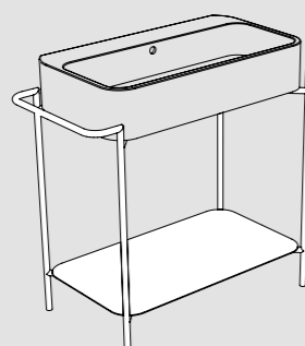
S868007 struttura_frame R8680 ripiano_shelf 90x45xh90 cm
